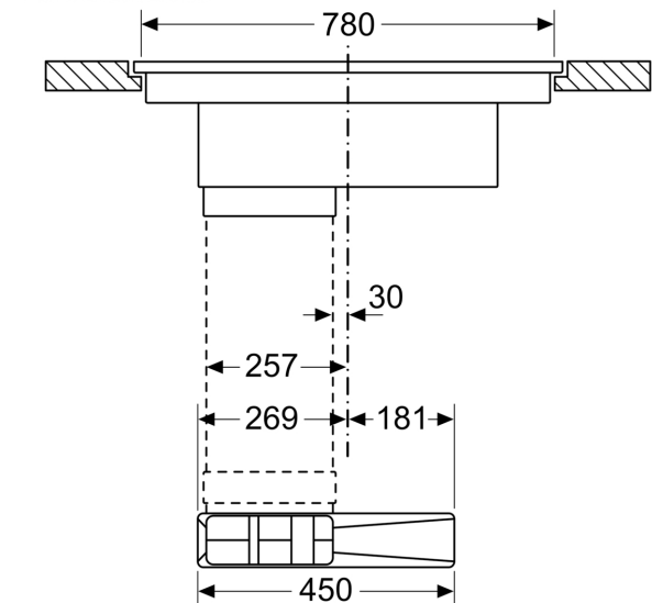
Maße in mm Vorderansicht
