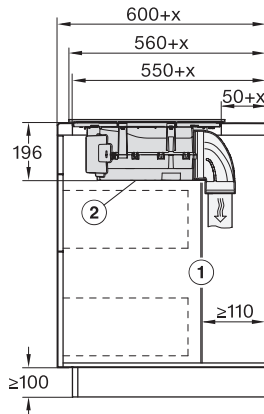
KMDA7272FL, KMDA7473FL – Skizze Seitenansicht aufliegend+X
