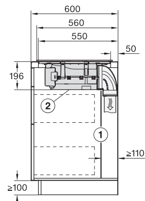
KMDA7272FL, KMDA7473FL – Skizze Seitenansicht aufliegend
