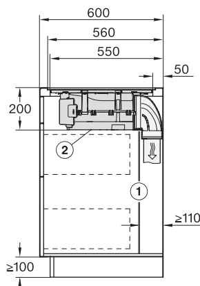
KMDA7272FL, KMDA7473FL – Skizze Seitenansicht flächenbündig
