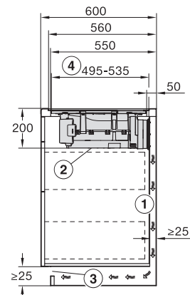
KMDA7272FL, KMDA7473FL – Skizze Seitenansicht flächenbündig, Plug&Play
