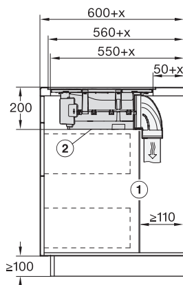
KMDA7272FL, KMDA7473FL – Skizze Seitenansicht flächenbündig+X
