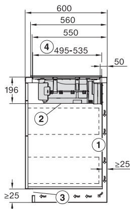
KMDA7272FL, KMDA7473FL – Skizze Seitenansicht aufliegend, Plug&Play
