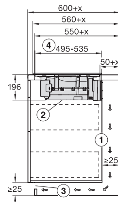
KMDA7272FL, KMDA7473FL – Skizze Seitenansicht aufliegend+X, Plug&Play
