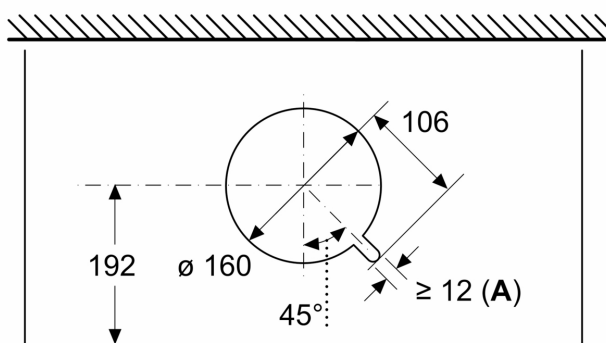
A: Kabeldurchführung
