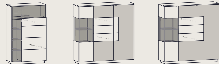
SIG-153130* B 92,8 | H 148,2 T 42
