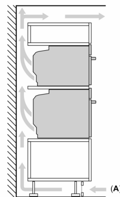
Einbau von zwei Geräten übereinander
